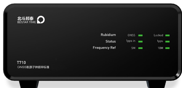
T710 前视图
